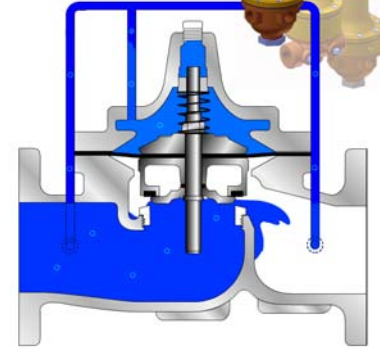
Modulierendes Kontrollventil
